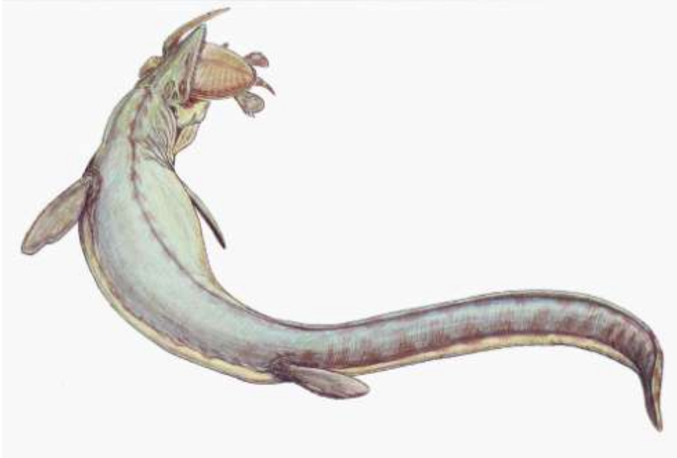
Mosasaurus
