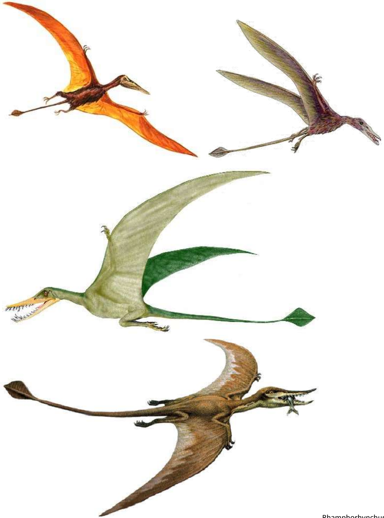
Rhamphorhynchus
