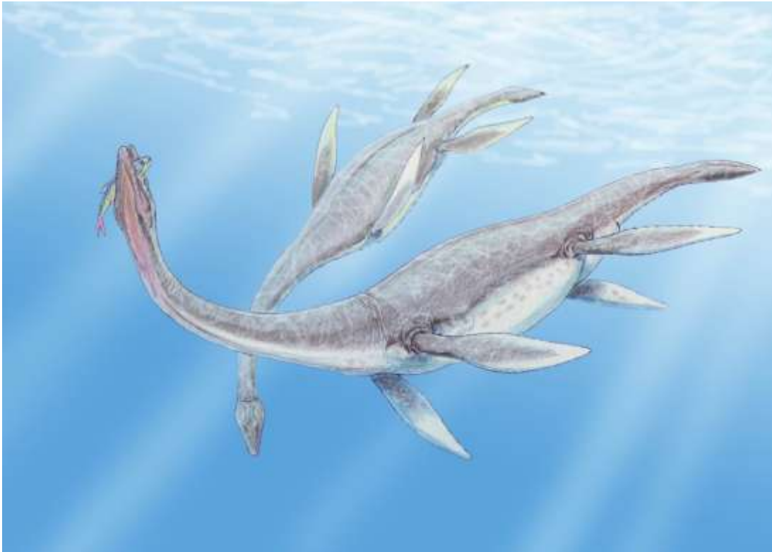
Plesiosaurus
